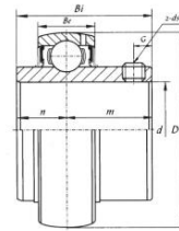
UCX00 (medium-duty)
