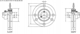
带冲压圆形密封外球面轴承
