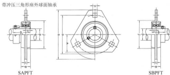
带冲压三角形座外球面轴承
