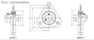
带冲压三角形座外球面轴承
